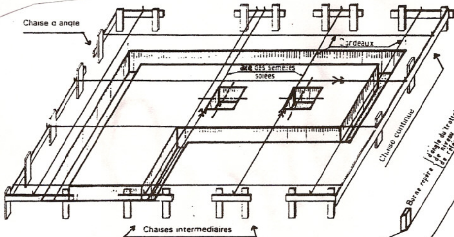
② Implantation d'un pavillon (chaises et cordeaux) Murs extérieurs et semelles isolées
