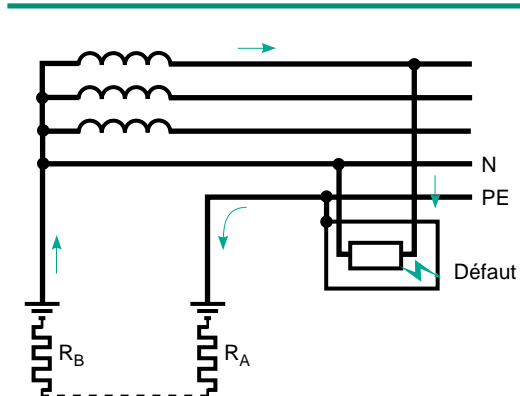
Fig. 7 : schéma TT.
