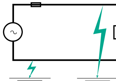
Défaut double le fusible fond si défauts francs
