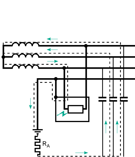
Fig. 8 : schéma IT.
